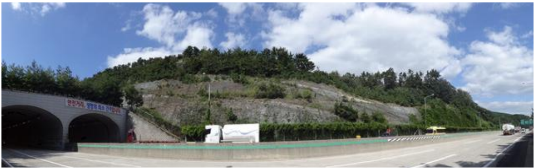
절토사면-부산포항선 STA.16+200~16+646(부산)
